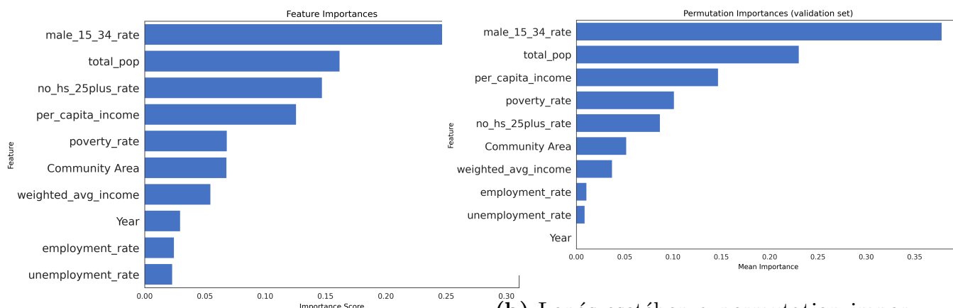
(b) Lopás esetében a permutation importance értékek
