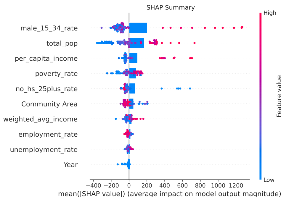
23. Ábra: Lopás esetében a feature importance értékek
