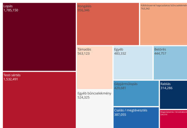
6. Ábra: Chicago bűnesemények típusai és gyakorisága
