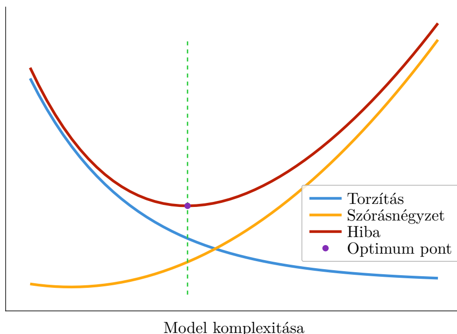
1. Ábra: Torzítás-szórásnégyzet kompromisszum illusztrációja
