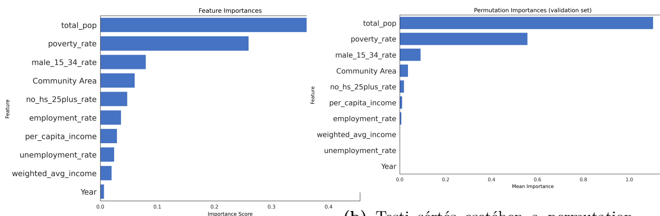
(b) Testi sértés esetében a permutation importance értékek
